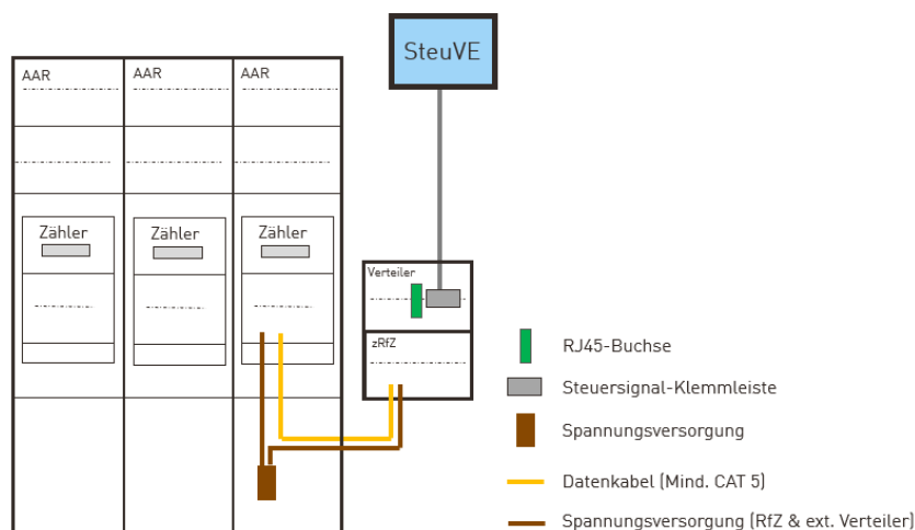
Abbildung 3: Vorbereitung Steuerung über einen externen Verteiler
